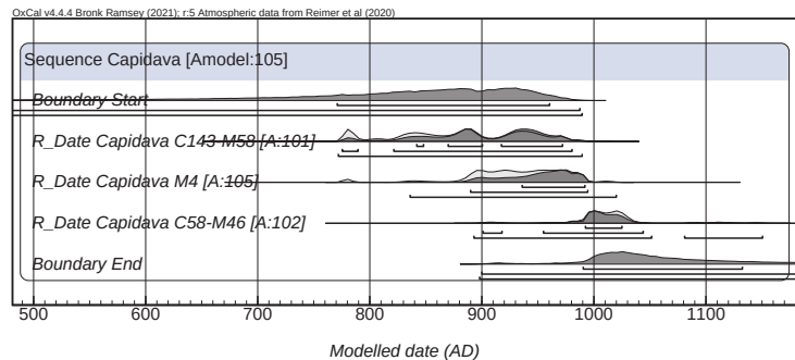
Figura 1. Analizele combinatorii ale probelor ^{14}\text{C} de la Capidava
