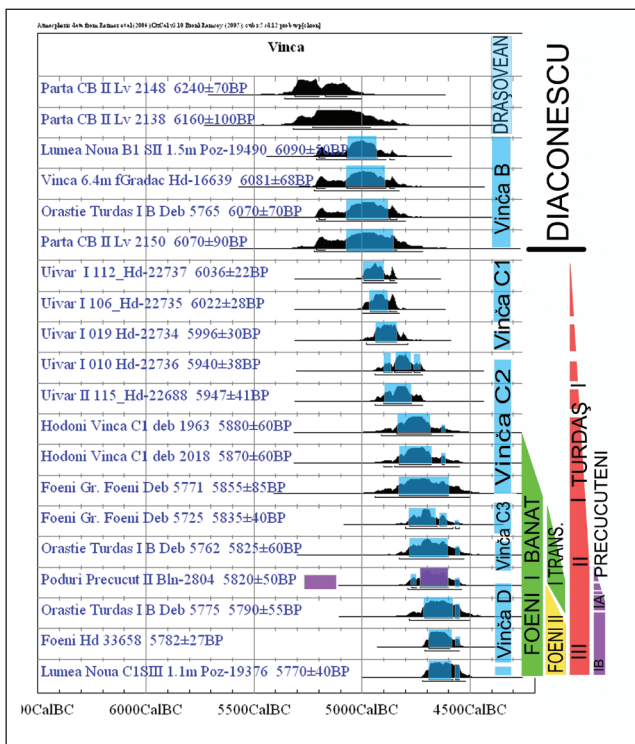
Fig. 34. Datele C14.
